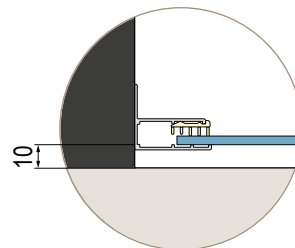
2. ábra Oldalfal
