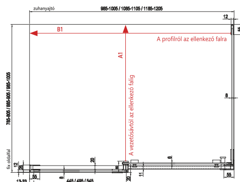
Zuhanyfolyókás telepítési segédlet
